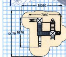
5448 ДЕТСКИЙ ИГРОВОЙ КОМПЛЕКС "ШАХМАТЫ"
