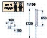
4295 СТОЙКА ДЕКОРАТИВНОГО ОГРАЖДЕНИЯ
