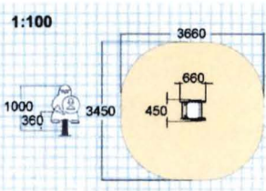
4162 КАЧАЛКА НА ПРУЖИНЕ "БОГАТЫРЬ"
