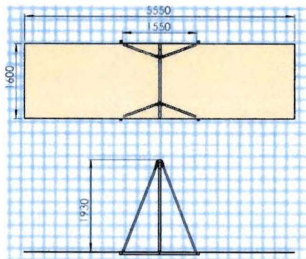
4154 РАМА КАЧЕЛИ НА МЕТАЛЛИЧЕСКИХ СТОЙКАХ
