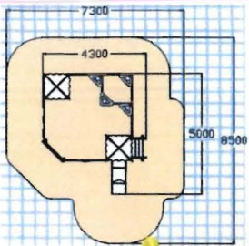
4287 ПЕСОЧНЫЙ ДВОРИК С ГОРКОЙ "ШАХМАТНЫЙ КЛУБ"
