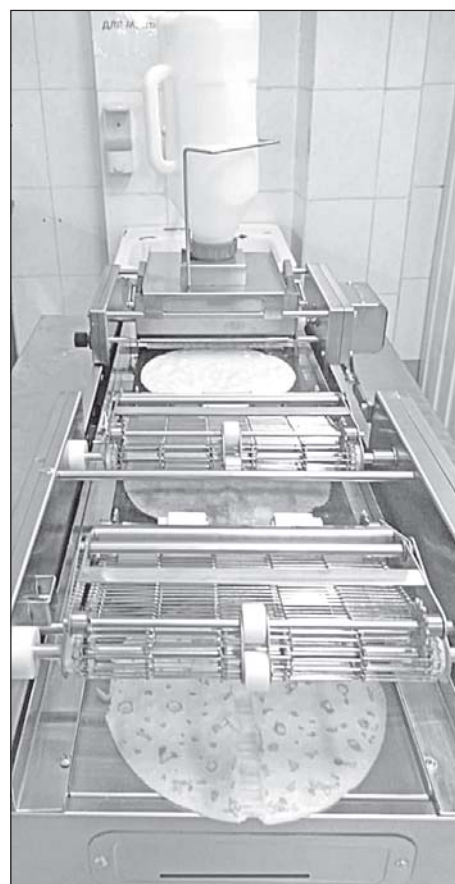
■ Блинный аппарат.
